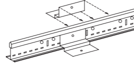
Универсальная клипса крепления перегородок, используемая с подвесной системой Prelude 15 или Prelude 24
