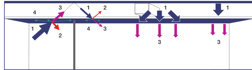
ПОГЛОЩЕНИЕ ИЗОЛЯЦИЯ (соседние помещения) ИЗОЛЯЦИЯ (звуки, идущие из потолочной пазухи) 1 Изначальный звук 2 Отраженный звук 3 Передающийся звук 4 Поглощенный звук 1-2 Звукопоглощение
